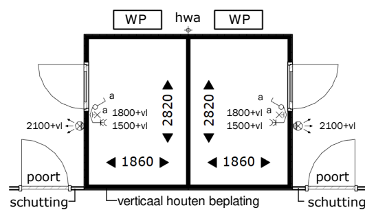
begane grond
