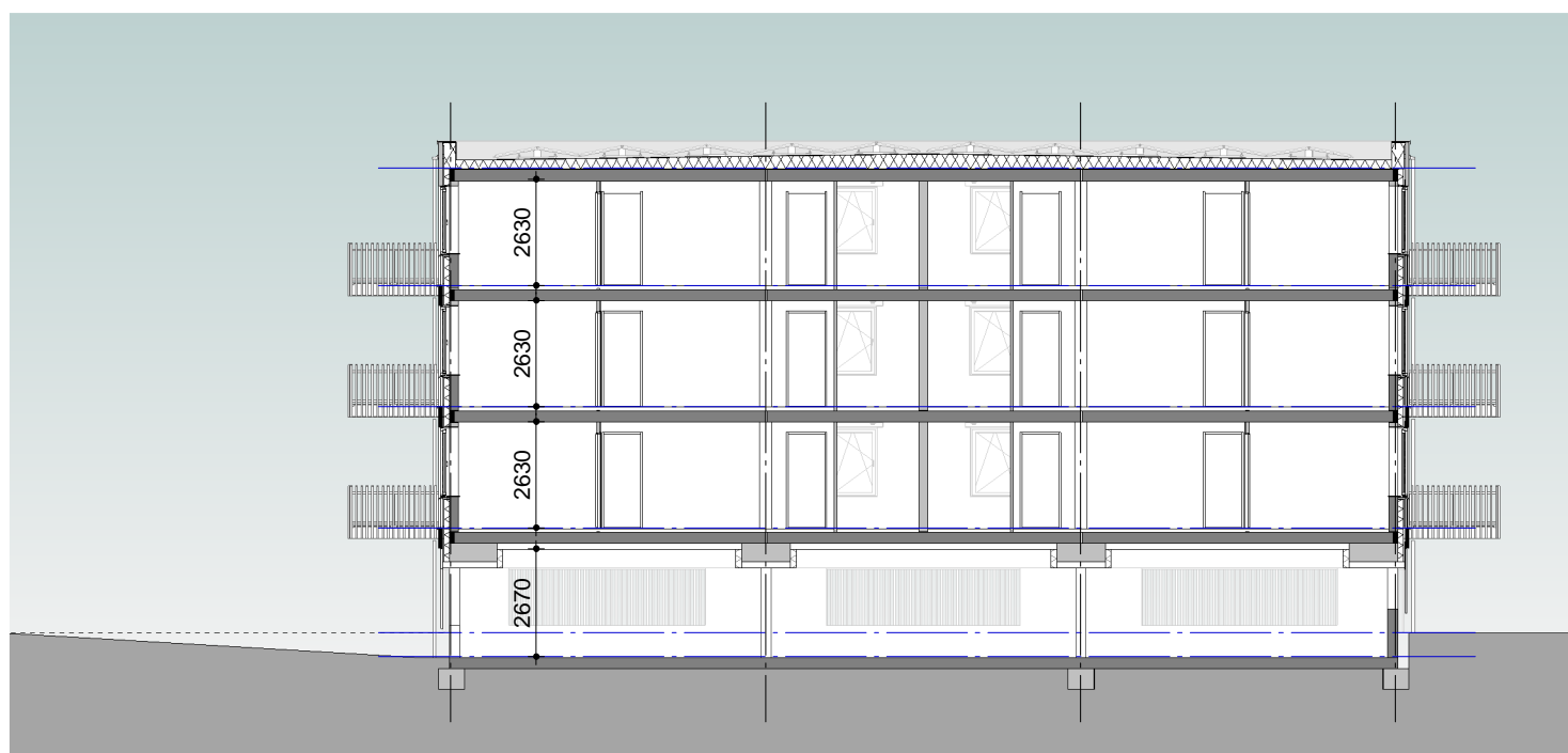
Doorsnede D
