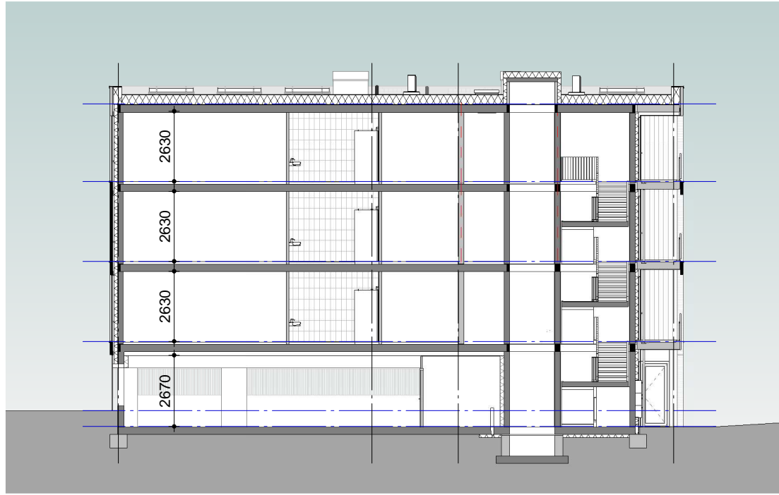
Doorsnede A
